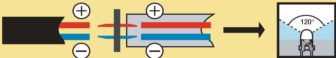
Соединение светодиодных светящихся трубок
